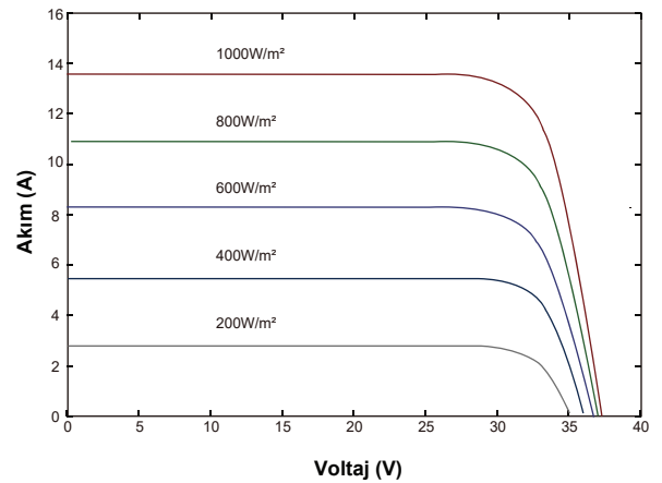
Akım - Voltaj Grafiği (CWT405-108PM10)
