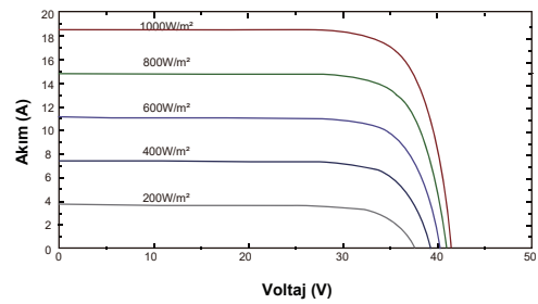
Akım - Voltaj Grafiği (CWT540-108PMB12)
