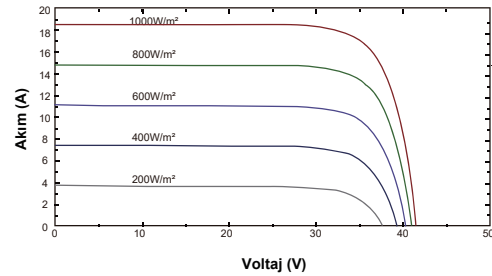
Akım - Voltaj Grafiği (CWT540-108PMBS12)
